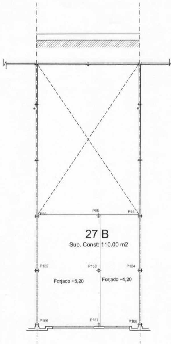
DISTRIBUCION PLANTA ALTA
